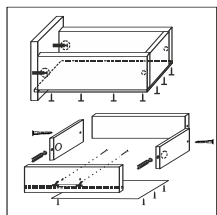
Сборка ящиков
