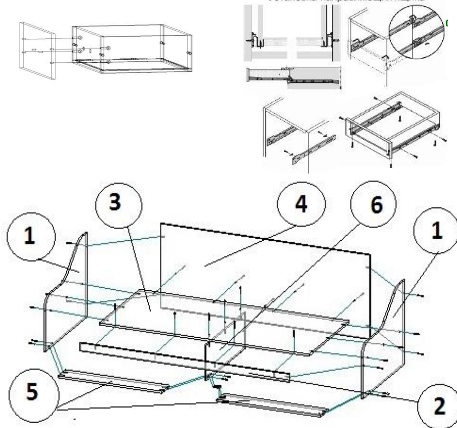
Установка направляющих ящика
