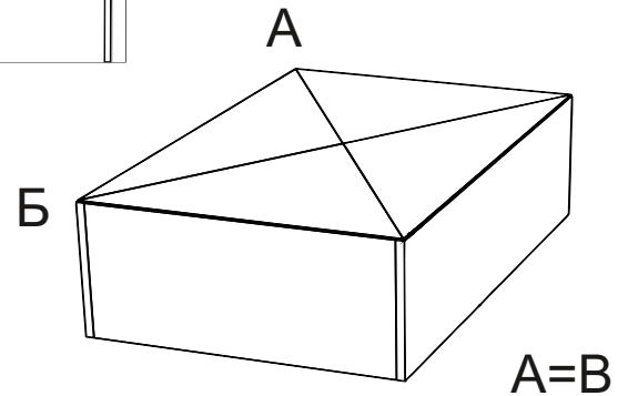
Проверка диагонали
